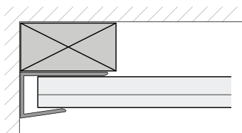
FCD202 Universal Edge Trim
